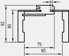
Przekrój ORB 075
