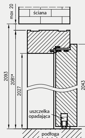
Ościeznica drewniana do drzwi Athos z uszczelką opadającą*
