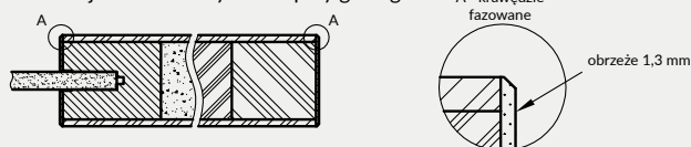
Przekrój ramienia skrzydła bezprzylgowego
