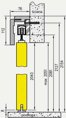
NS - przekrój pionowy
