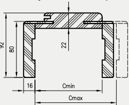
Przekrój poziomy OR/ORC
