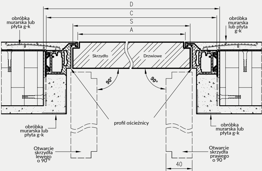
Przekrój poprzeczny drzwi Sara Eco 2 z odwróconą przylgą - otwierane do wewnątrz
