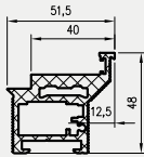
Profil do drzwi z odwróconą przylgą otwieranych do wewnątrz
