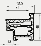
Profil do drzwi bezprzylgowych otwieranych na zewnątrz
